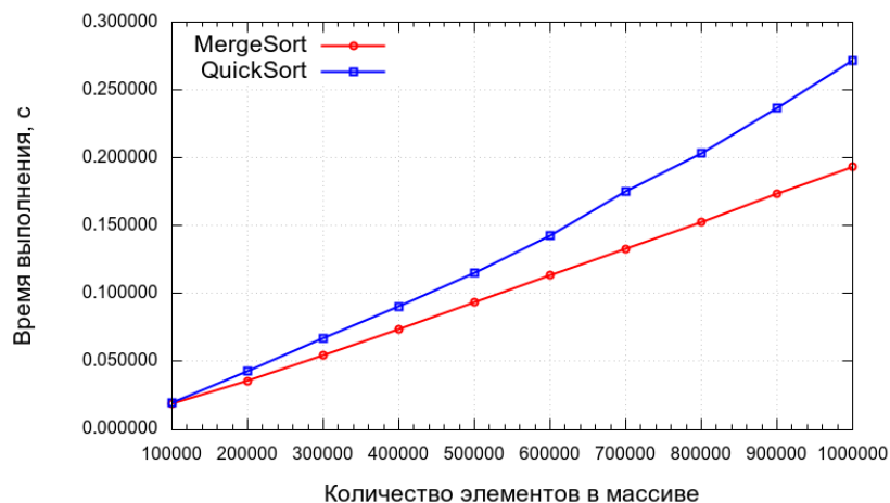
Рис. 1. Зависимость времени выполнения алгоритмов MergeSort и QuickSort от количества элементов в массиве
